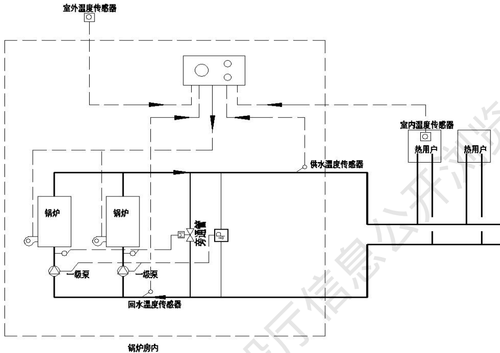
图4 燃气锅炉和用户侧均变流量运行的一级泵系统示意图
