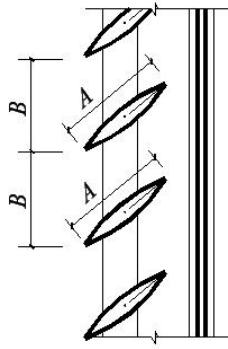
图 D.0.1-4 横百叶挡板式外遮阳的特征示意图
