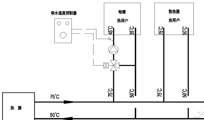
图 5 同一热源服务于不同水温需求热用户时的混水泵供热方式示意图
