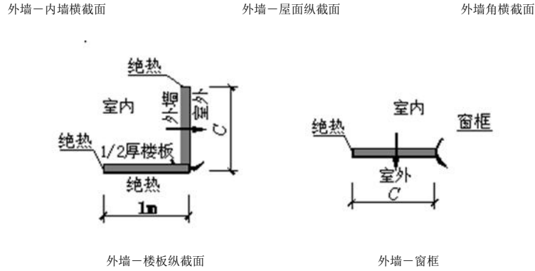
图 B.0.5 墙面典型结构性热桥截面示意图
