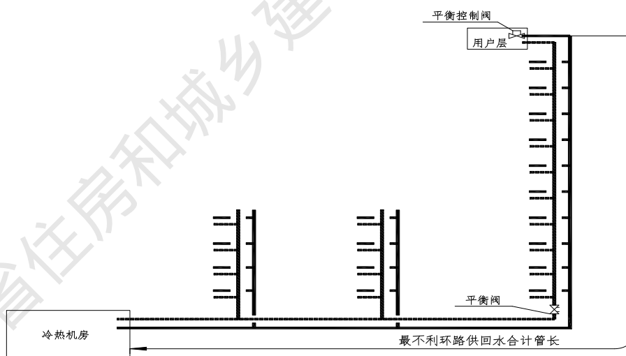
图 6 从冷热机房至该系统最远用户的供回水主干管长度 \Sigma L 示意图
