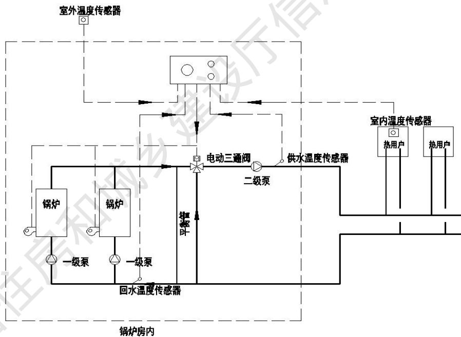
图 1 燃气锅炉二级泵混水系统示意图
