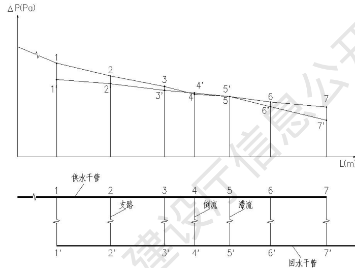
图 8 同程系统布置及管路压力分析图
