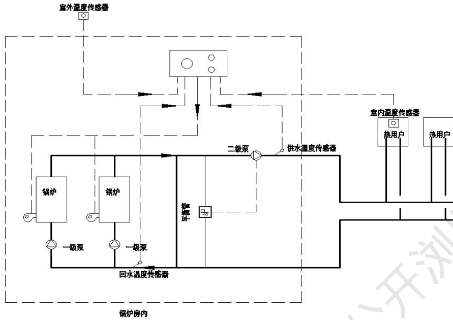
图 2 燃气锅炉定流量用户侧变流量运行的二级泵系统示意图
