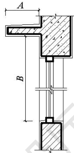
图 D.0.1-1 水平式外遮阳的特征值示意图
