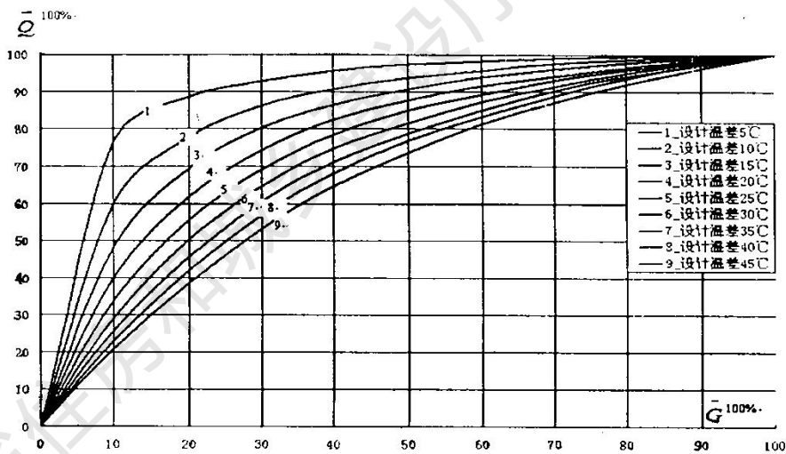
图7 散热器流量和散热量的关系曲线
