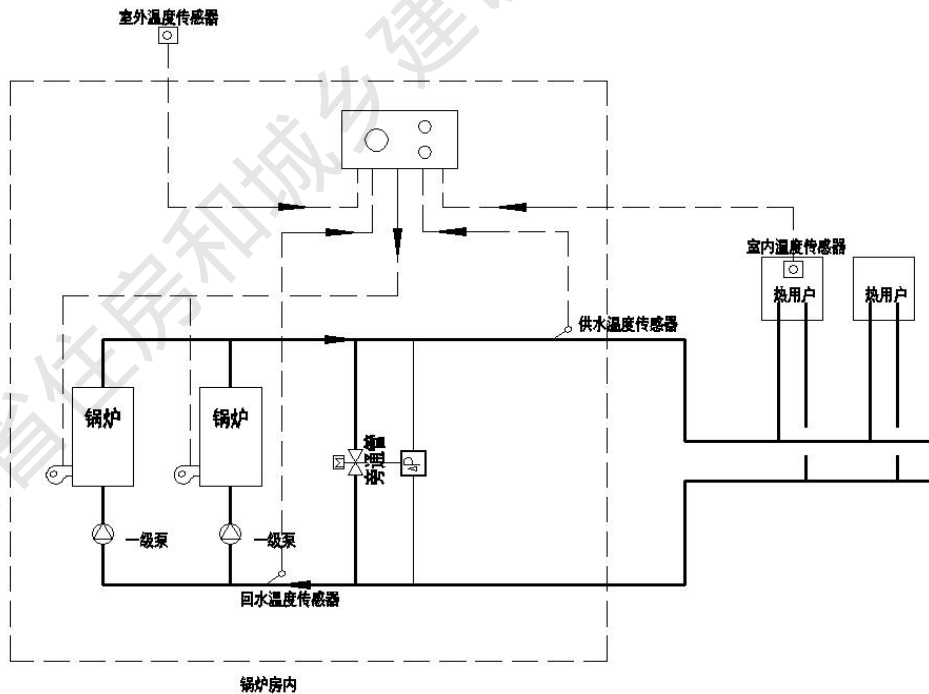
图 3 燃气锅炉定流量用户侧变流量运行的一级泵系统示意图
