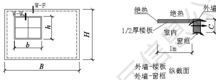
图 B.0.6 墙面平行热桥示意图
